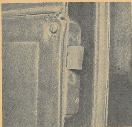
Palen i en dørlås er her blevet fuldkommen deformeret, fordi håndtagsmekanismen har manglet olie igennem lange tider. Går mekanismen trægt, skal palen påvirkes altfor voldsomt for at døren kan smækkes. Ved de gentagne hårde lukninger er hele dørlåsen gået løs, bemærk den nederste skrue, der er på »dinglestadlet».
