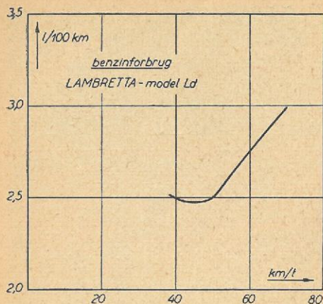
Benzinforbruget for Lambretta er ret normalt ved de laveste hastigheder, men stiger ret kraftigt efterhånden som hastigheden sættes op.
