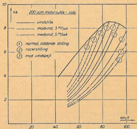
Effektdiagram for en tilfældigt valgt motorcykel på 200 ccm — motoren udvikler 8,5 hk ved 4150 omdr. min. Øverst på figuren ses motorens hestekraftkurve ved kørsel med gashåndtaget i bund, og endvidere er indtegnet de forskellige kurver for køremodstanden i de ni gennemregnede tilfælde. Se iverigt teksten.
