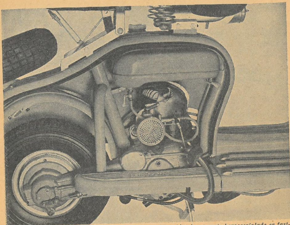
*Karosseriet på Lambretta er udformet som tre stykker, idet den øverste karosseriplade er fastmonteret til stelkonstruktionen, medens de to sideplader er aflagelige, således at man uhindret kan komme til motoraggregatet. Umiddelbart over motoren ligger benzintanken, man ser benzinhænan, der er udformet som en almindelig tregangshane. Karburatoren er monteret med et luftspjæld, som skydes ned ved hjælp af en trykslang på karburatoren. Bemærk tørrigt bundspjæld, der er ført helt tilbage til baghjulet, og således tjener som fodbrædd for bagsædepassageren. Stellets udformning giver mulighed for at montere en sving sadel til bagsædepassageren, og som det fremgår af illustrationen, har denne sving sadel en meget stor affjedringsbevægelse. De to sadler er iøvrigt næsten lige høje.
