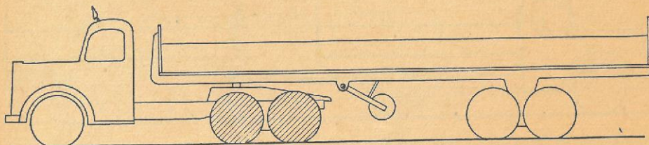
3-akslet lastbil med dobbeltakslet sættevogn. Ved køretøjer af denne art kan man — indenfor den gældende lovgivning — opnå den størst mulige nyttelast på et enkelt lad. Se tørrikt teksten.
