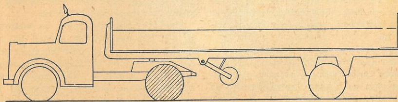
2-akslet lastbil med 1-akslet sættevogn — sættevognen hviler med sin forreste ende ved hjælp af et enkelt, svært dimensioneret kugleled på en skammel på motorvognens chassissamme — ved frakobling af sættevognen hviler dennes forreste ende på de viste, nedfældbare støttehjul.
