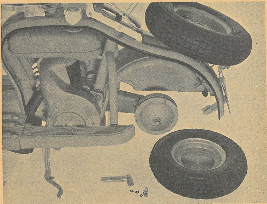
Fra denne side ses blæskappen, der leder køleluften fra svinghjulsblæseren op om cylinder og topstykke. Som det fremgår af illustrationen, er baghjulet aftageligt som på en bil, blot ved at løsne tre møtrikker. Påfyldningsslutsen til benzintanken er let tilgængelig, og man vil endvidere se, at der over baghjulet er monteret en bagskærm, således at vejsnavs ikke kommer direkte op til karosseripladen. De to aftagelige sidestykker er monteret i gummitlister. Umiddelbart bag blæskappen ser man vridearmen til torsionsfjederen.
