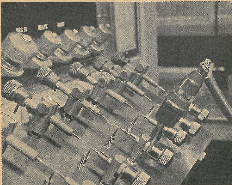
Gnistforstærkeren monteret i prøveanlægget på Lucas værkstedet, hos fa. Axel Ketner. Det her viste gnistgab er 11 mm, og med gnistforstærkeren indskudt mellem højspændingsledningen og gnistgabets var gnisten regelmæssig, medens gnisten blev uregelmæssig så snart gnistforstærkeren fjernedes.
