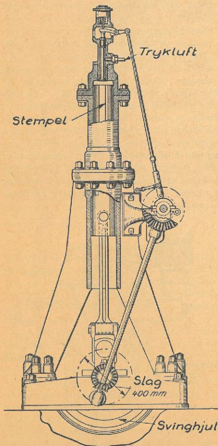
Skematisk tegning af Diesel's første forsøgsmaskine — der var ingen vandkappe omkring cylinderen, og brændstet blev sprøjtet ind gennem en ventil i topstykket ved hjælp af trykluft fra en kompressor uden for selve motoren. Kompressionslufttrykket var 40—45 at., brændstet petroleum og forbruget ca. 240 g/hk. Den ukølede cylinder tillod selvfølgelig kun ganske kort tids drift under belastning.
