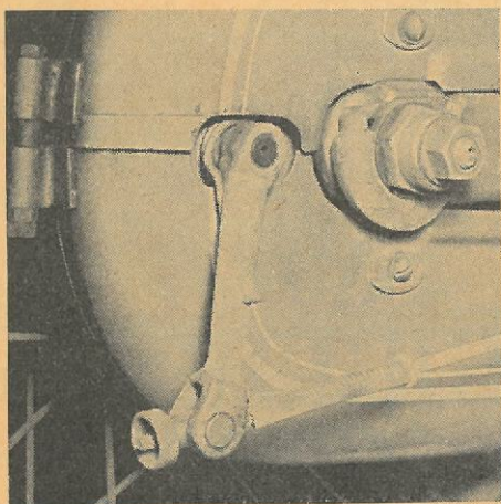
Mellem bremsestang og bremsearm på en motorcykel er der altid et led, der bør smøres. Naturligvis vil bremsen fungere udmærket, hvodenten dette led er smurt eller ikke, men rusttæring og slid vil efterhånden gøre forbindelsen løsagtig og raslende.
