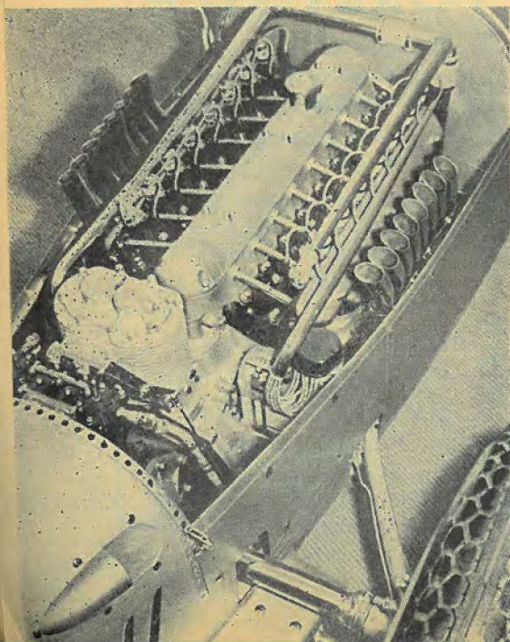
Auto-Union Racermotor af Aargang 1935. Bemærk de skraatliggende Stødstænger til Udblæsningsventilerne.
