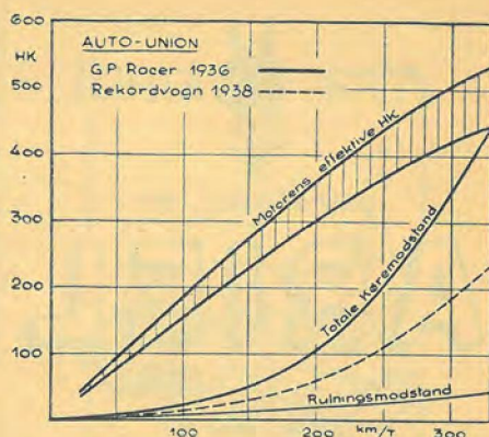
Fig. 3. Effektdiagram for Auto-Union Grand Prix Racer, Aargang 1936. Det skraverede Areal fremstiller Tabet i Hestekraft mellem Motorens Købingsflange og Vejbanen. Den punkterede Kurve giver til Sammenligning Køremodstanden for 1938 Rekordvognen med Strømliniekarosseri.
