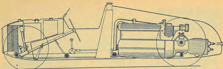
Fig. 1. Skematisk Snit igennem Auto-Union Racer af Aargang 1934. Motoren hælder 2° Grader bagover, saaledes at Akslen til Gearkassen kan passere under Differentiallet.
