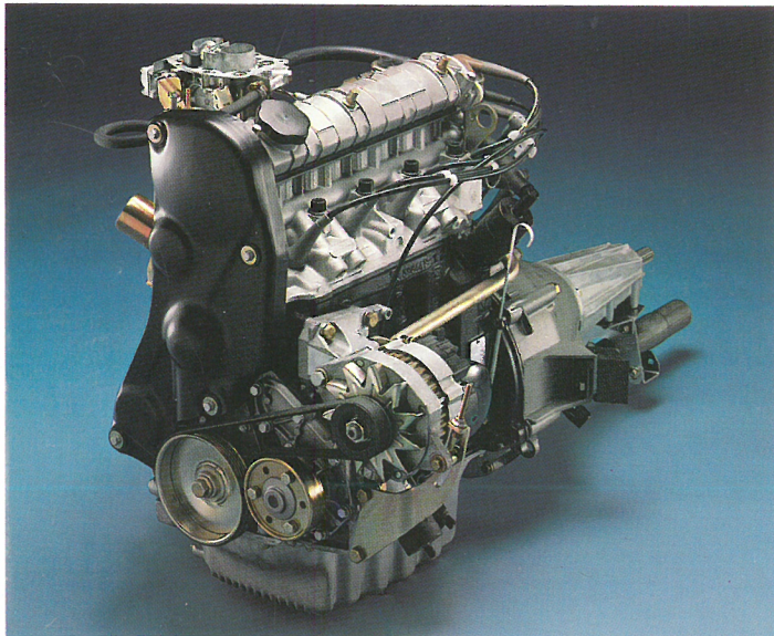
Volvo 340 GL 1,7 liter motor.
