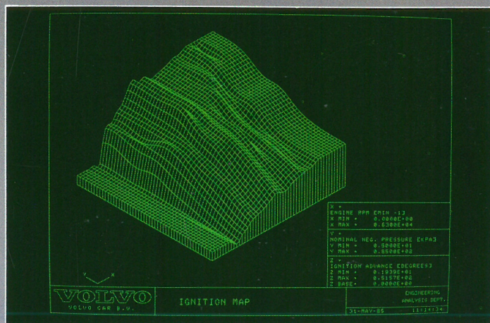
Diagram over tændingstidspunkter i det elektroniske tændingssystem.
