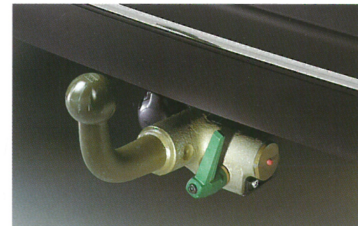
Et aftageligt afhængertræk, godkendt efter ISO og DIN specifikationerne og grundigt testet af Saab. Det er konstrueret, så det presses nedad og væk fra benzintanken i tilfælde af kollision bagfra.
