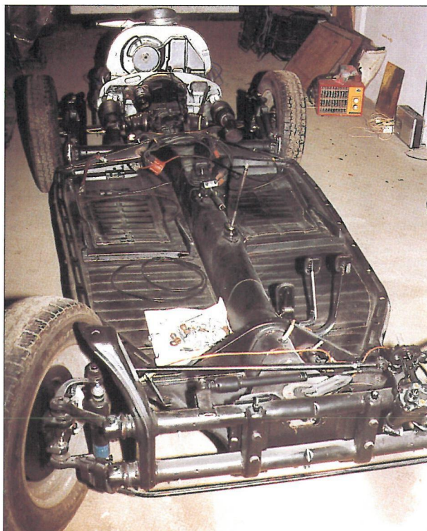
Platformen under genopbygning. Bunden er sandblæst og metalliseret. Nye bremse- og benzindrør m.v. er lette at installere her. Motor er hovedrepareret, og alt kontrolleret inden samling.
